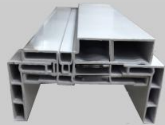
วงกบ UPVC 9.5cm. + ซีบ
