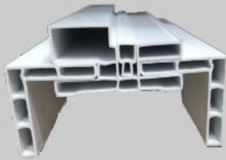
วงกบ UPVC 7cm. + ซีบ
